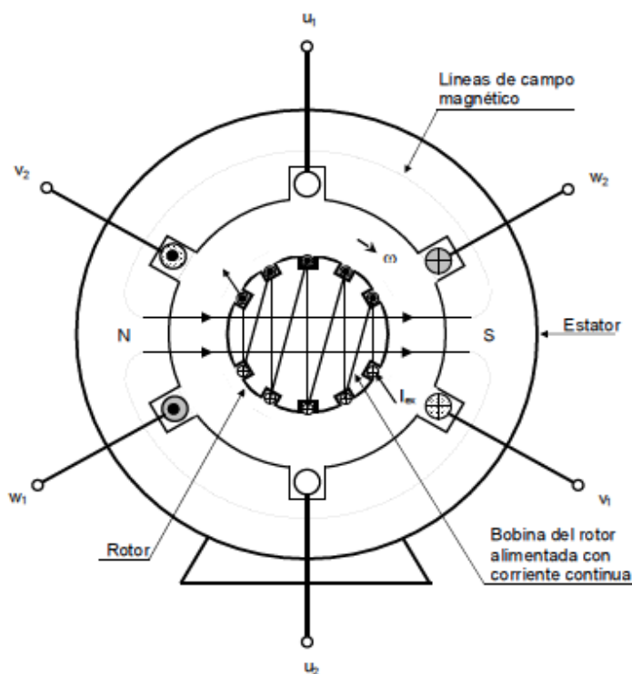
Esquema de un generador trifásico síncrono
