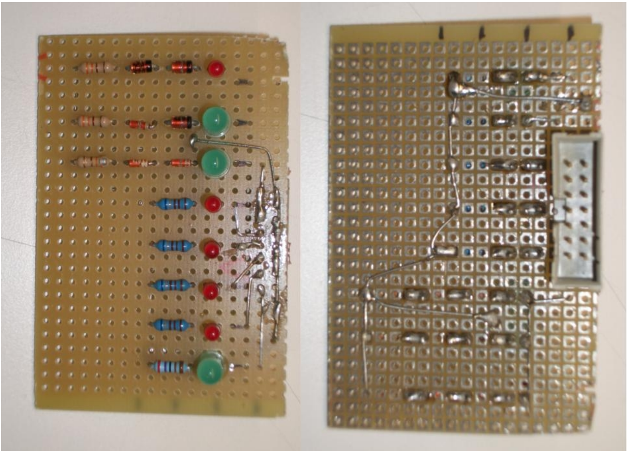
Panel indicador de estado
