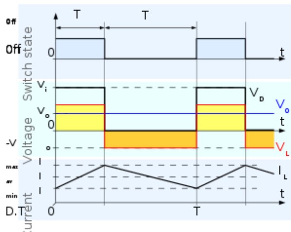
Evolución de las tensiones y corrientes en conducción continua de un buck
