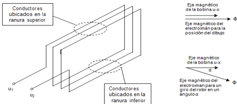
Esquema de la bobina U
