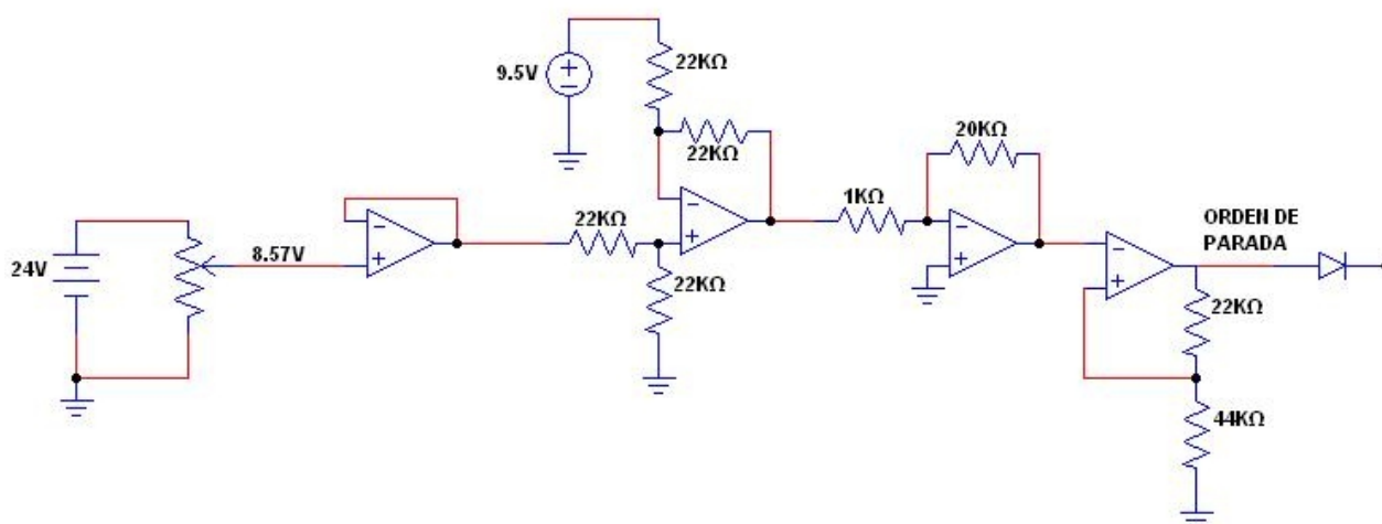
Orden de parada por sobrecarga de las baterías
