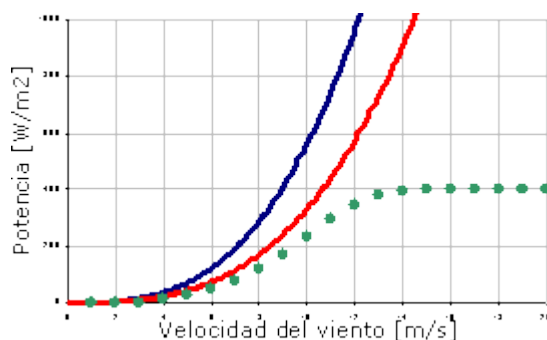
Potencial extraíble por metro cuadrado de área cubierta por el rotor.
