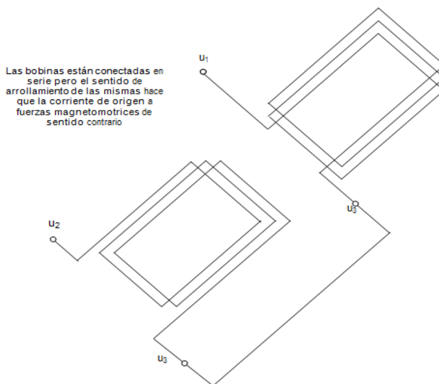
Esquema del bobinado para una fase
