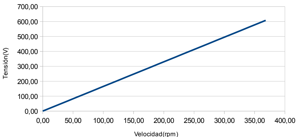
Valor de la tensión rectificada en función de la velocidad
