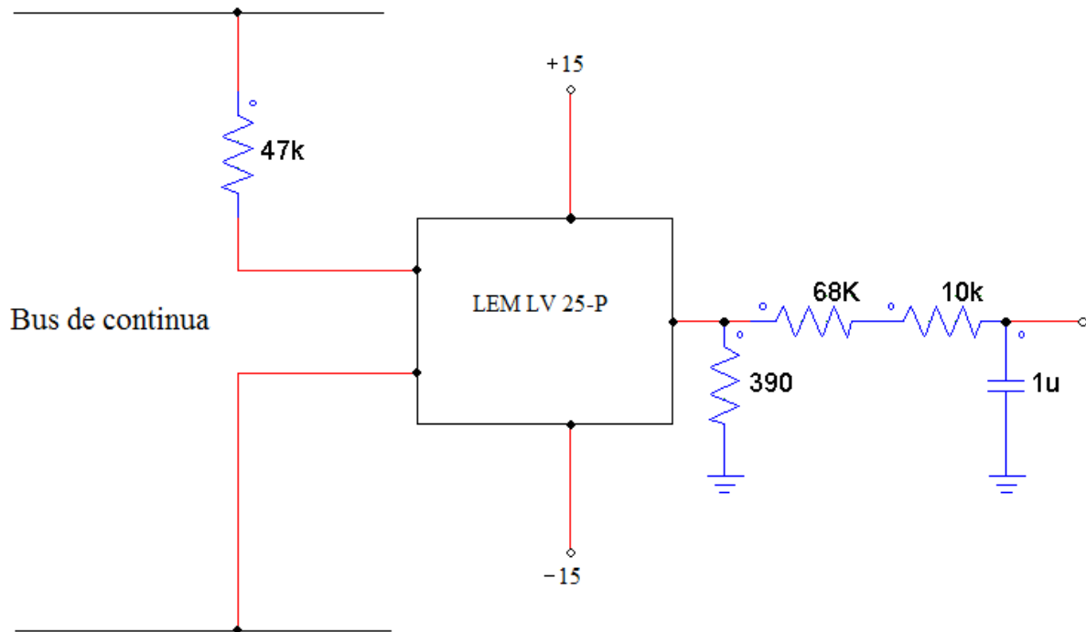
Transductor de tensión y filtro
